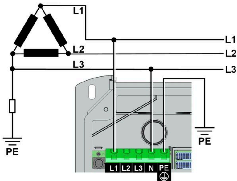
Tilkobling til et 3-leders IT-system.
